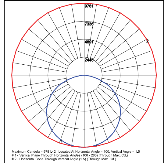
EESCP20QF1X186U 5KC Type V
