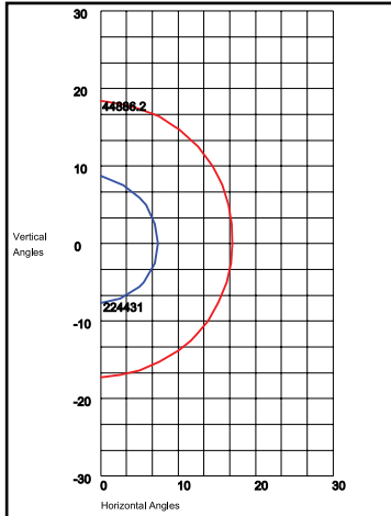
EES-SP52Q33536U5K 16°H x 16°V Beam, NEMA 3H x 3V
